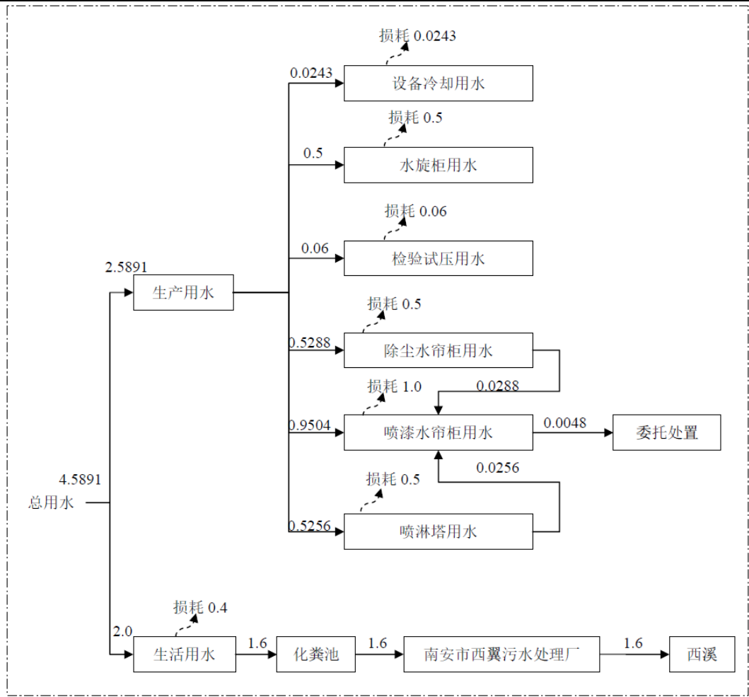
图 2.6-1 项目水平衡图 单位: t/d
