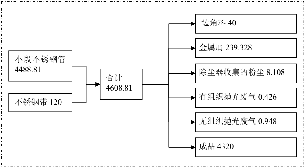
图 2.7-1 项目物料平衡图 (单位: t/a)
